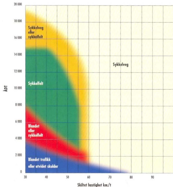
Figur 11. Valg av sykkelløsning avhengig av trafikkmengde (ÅDT) og skiltet fartsgrense. (Statens vegvesen, 2003)
